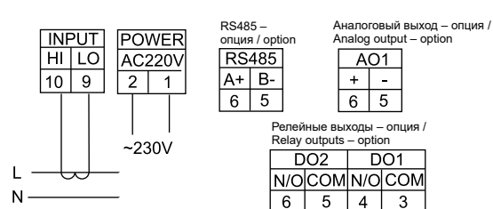
Схема подключения 1-ф. амперметра при I > 5 A
