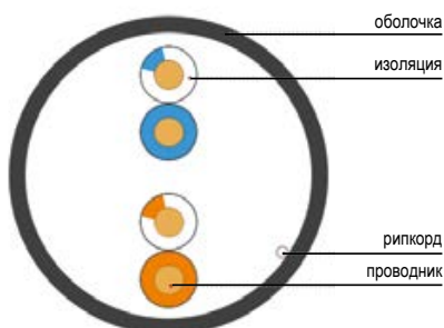
Конструкция кабеля типа U/UTP (количество жил 2 \times 2 )
