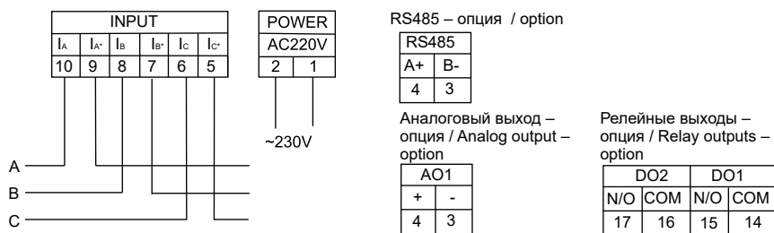
Схема подключения 3-ф. амперметра при I \leq 5 A
