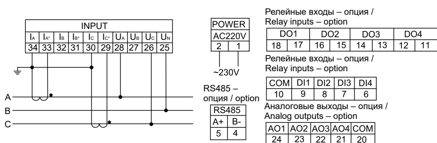
Схема подключения мультиметра к трехпроводной сети при I > 5 A, U \leq 600 В
