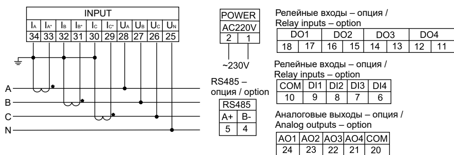
Схема подключения мультиметра к четырехпроводной сети при I > 5 A, U \leq 600 В
