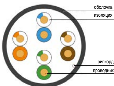
Конструкция кабеля типа U/UTP (количество жил 4 \times 2 )
