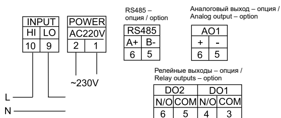
Схема подключения 1-ф. амперметра при I \leq 5 A
