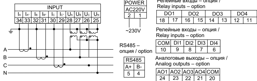
Схема подключения мультиметра к четырехпроводной сети при I>5 A, U>600 В
