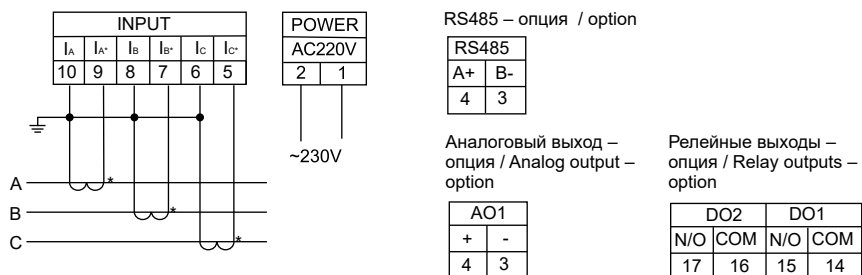
Схема подключения 3-ф. амперметра при I > 5 A
