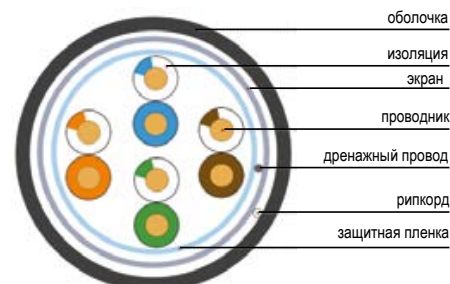
Конструкция кабеля типа F/UTP (количество жил 4 \times 2 )
